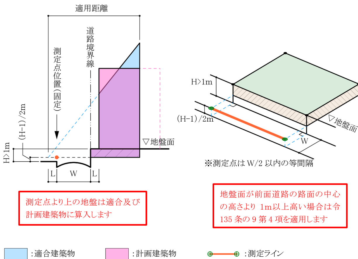
図 7-2-1-8 地盤面が測定点の高さより高い場合
