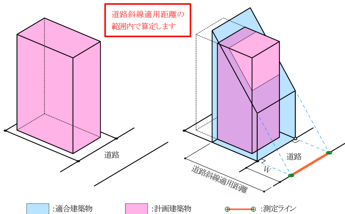
図 6-2-1-1 道路高さ制限における天空率算定領域
