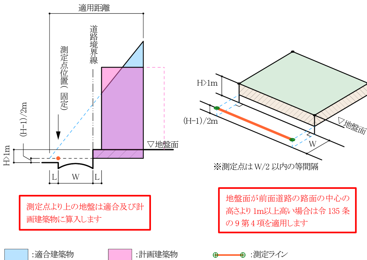
図 6-2-1-8 地盤面が測定点の高さより高い場合
