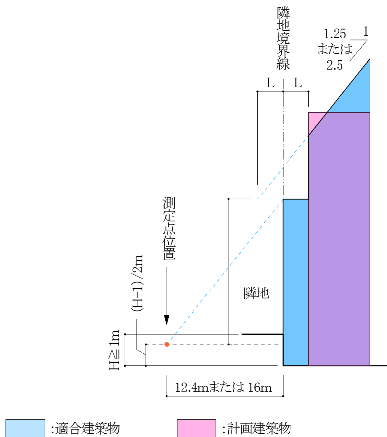
図 6-2-2-5 敷地が公園・広場・水面等に接している場合
