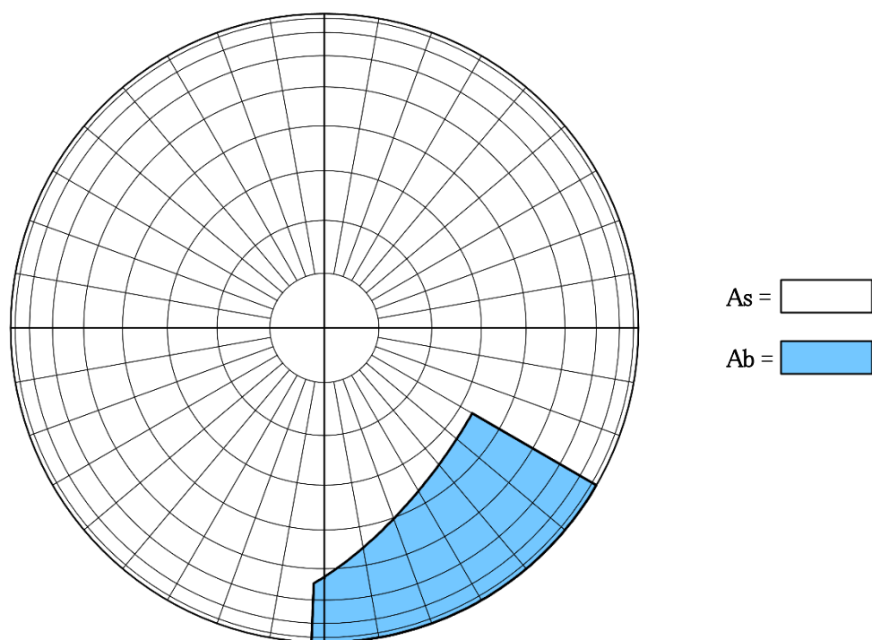
図 6-1-1-1 天空率
