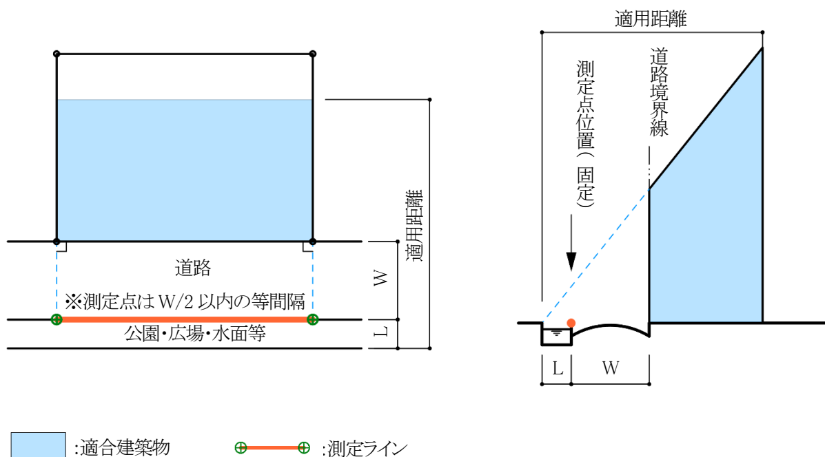
図 6-2-1-8 地盤面が測定点の高さより高い場合
