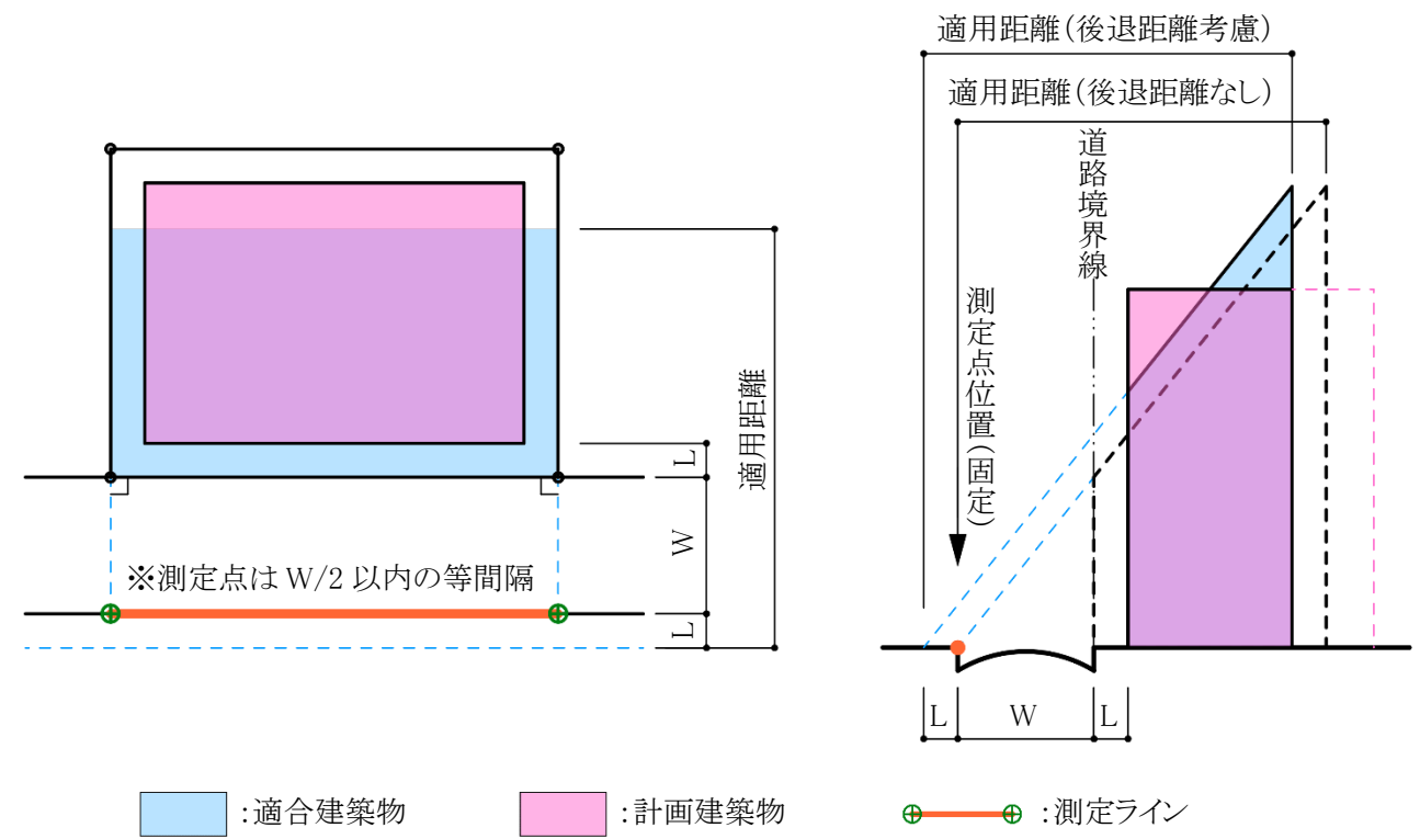
図 7-2-1-2 後退距離による適合建築物の違い
