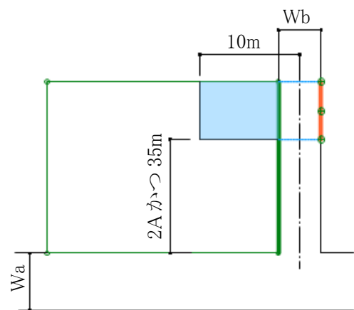
天空率算定領域 No3
