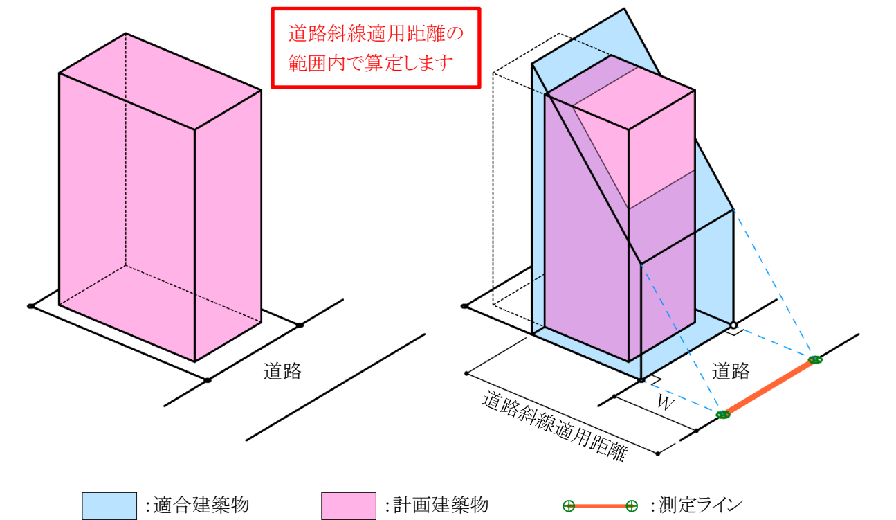
図 7-2-1-2 後退距離による適合建築物の違い
