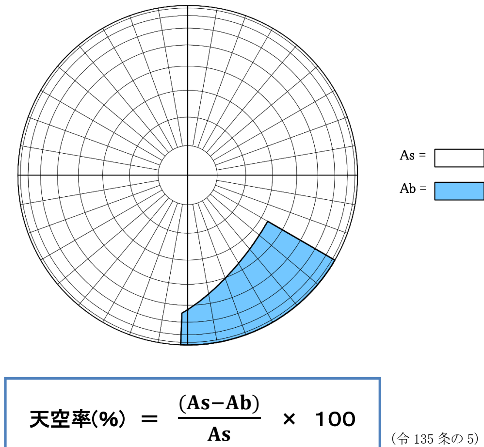
図 7-1-1-1 天空率
